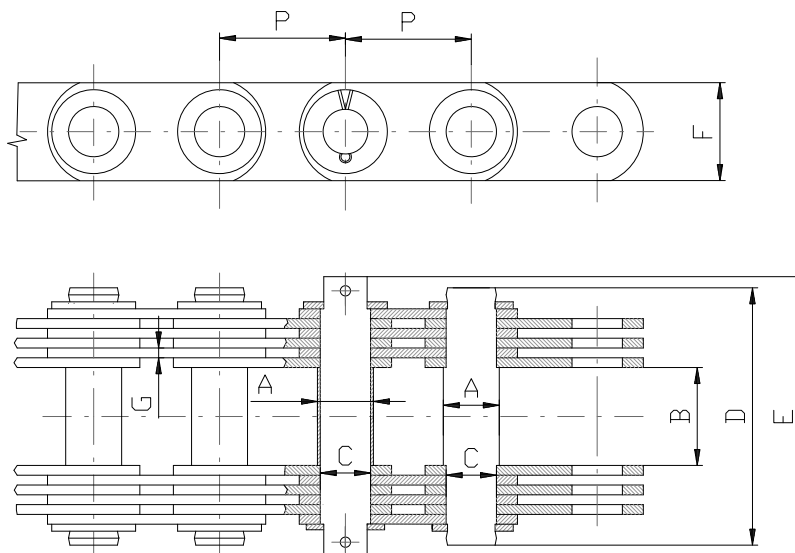
Gallové řetězy DG70 - DG120
