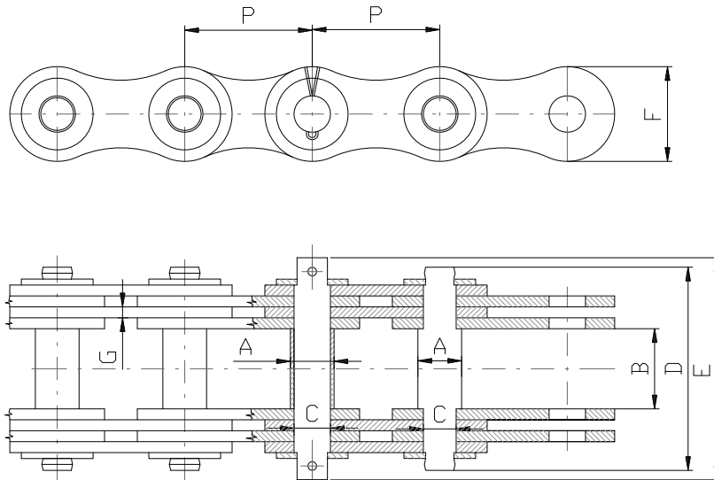
Gallové řetězy DG50 - DG60
