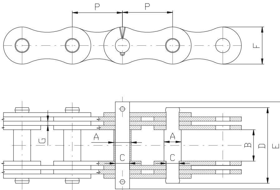
Gallové řetězy DG25 - DG45
